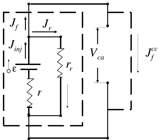
Figura 3 - Os elementos físicos do circuito interno de uma CSNS são: resistência interna ( r ), força eletromotriz de injeção de elétrons ( \varepsilon ) e resistência interna de recombinação ( r_r ).
