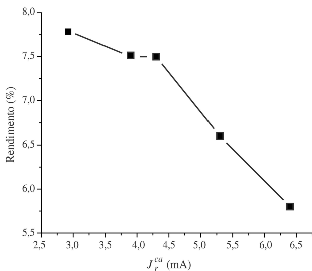
Figura 4 - Aumento na eficiência de uma CSNS, quando a corrente de recombinação interna J_r^{ca} diminui. Os valores foram obtidos a partir da Eq. (9), com os dados da Tabela 1 e atribuindo-se o valor de 1 V para a fem .
