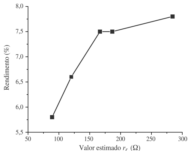
Figura 5 - Aumento na eficiência de uma CSNS quando a resistência de recombinação interna r_r aumenta. Os valores foram obtidos a partir da Eq. (10), da Tabela 1 e atribuindo-se o valor de 1 V para fem .
