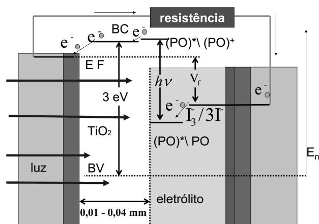
Figura 2 - Diagrama de energia de uma CSNS. O eletrodo negativo com TiO 2 é sensibilizado com um PO que ao receber luz, excita seus elétrons, (PO)*, e passa a injetá-los na BC do TiO 2 , deixando com isso, buracos em suas moléculas (PO) + . Os elétrons que vão para a BC do TiO 2 podem percorrer um caminho dentro desse semiconductor e chegar ao substrato saindo então da CSNS. Percorrendo um circuito externo os elétrons chegam ao eletrodo positivo com menor energia, onde completam o ciclo. Adaptado da Fig. 1 da Ref. [3].
