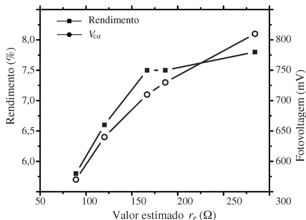
Figura 6 - Comparação entre a curva da fotovoltagem, V_{ca} , com a curva de eficiência em função da resistência interna de recombinação, r_r , em uma CSNS. Os valores foram obtidos fazendo uso da Tabela 1 e da Eq. (10), atribuindo-se o valor de 1 V para \varepsilon . O valor da eficiência é dado em termos percentuais. Observa-se um aumento na eficiência juntamente com a V_{ca} , quando ocorre também um aumento na resistência interna de recombinação.
