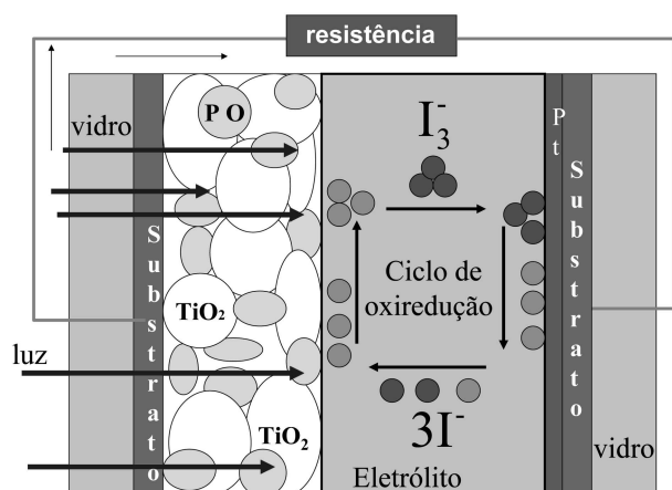
Figura 1 - Componentes de uma CSNS. A célula é composta de duas placas de vidro recoberto por um substrato condutor transparente de \text{SnO}_2 . Sobre lado condutor de uma dessas placas é depositado um filme de 10-40 \mu\text{m} de largura com \text{TiO}_2 , que é sensibilizado com PO formando assim o eletrodo negativo. Na outra placa é depositada uma fina camada de platina ou grafite que será o eletrodo positivo. A célula é preenchida com um eletrólito contendo íons de iodo e triiodeto. Também é mostrado de forma ilustrativa o ciclo de oxidação-redução dos íons de iodo, 3\text{I}^- em \text{I}_3^- .
