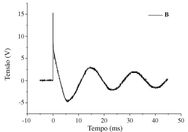
Figura 2 - Tensão nos terminais da bobina em função do tempo.
