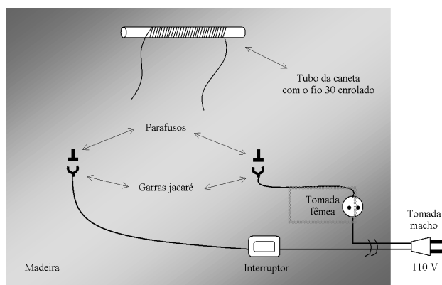
Figura 1 - Esboço do experimento.
