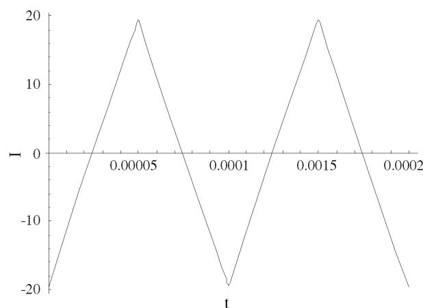
Figura 7 - Forma de onda da corrente em resposta a uma onda de tensão quadrada de frequência fundamental igual a 10 kHz. Para o cálculo da impedância foi levada em consideração a indutância externa.
