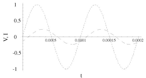
Figura 3 - Evolução no tempo da tensão com amplitude unitária e corrente (curva em traço largo) em um condutor filiforme retilíneo de um metro de comprimento e diâmetro 3 mm. Para o cálculo da impedância foi levada em consideração a indutância externa do fio. A corrente elétrica é expressa em kA.
