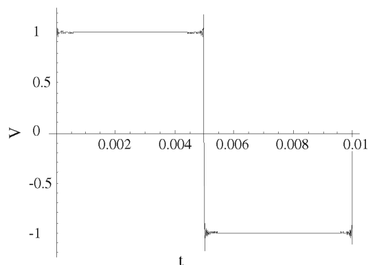
Figura 5 - Representação de uma onda quadrada de tensão com amplitude unitária e frequência fundamental f = 100 Hz.
