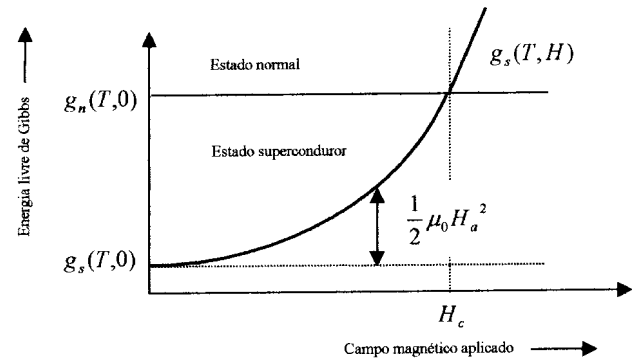
Figura 14: Efeito do campo magnético sobre a energia livre de Gibbs nas fases normal e supercondutora (figura retirada de Rose-Innes e Rhoderick, 1988).
