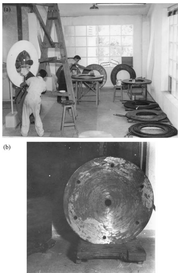
Figura 12 - (a) Panquecas do eletroímã com isolamentos rompidos; (b) polos enferrujados.
