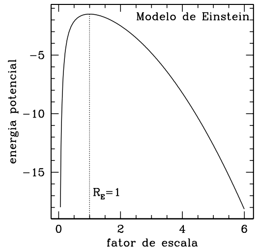
Figura 1 - Diagrama na forma da letra \Lambda : a energia potencial na analogia newtoniana do modelo estático de Einstein. Note que o ponto de equilíbrio em R = R_E é um ponto de equilíbrio instável. Uma pequena perturbação em R_E resultará no colapso do universo ou na divergência para R \rightarrow \infty .
