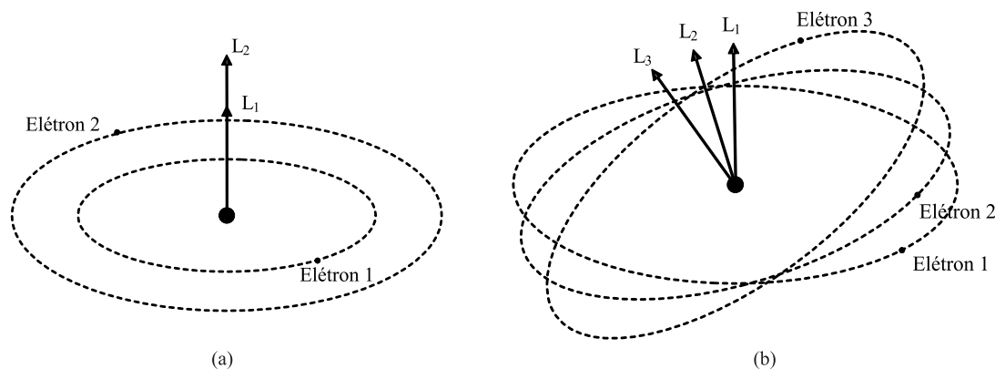
Figura 2 - (a) Modelo de Bohr; (b) Modelo de Sommerfeld.
