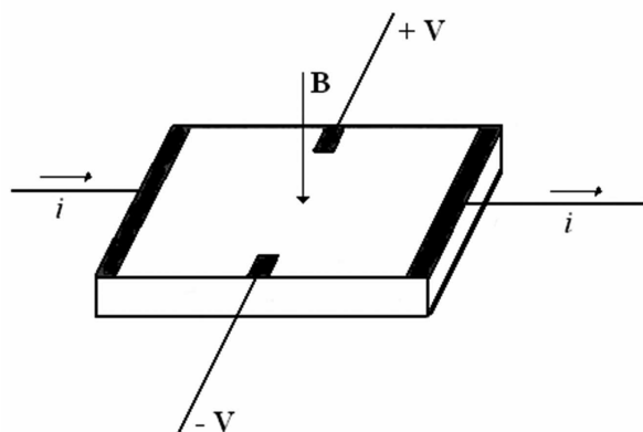
Figura 3 - Sensor de campo magnético baseado no efeito Hall.
