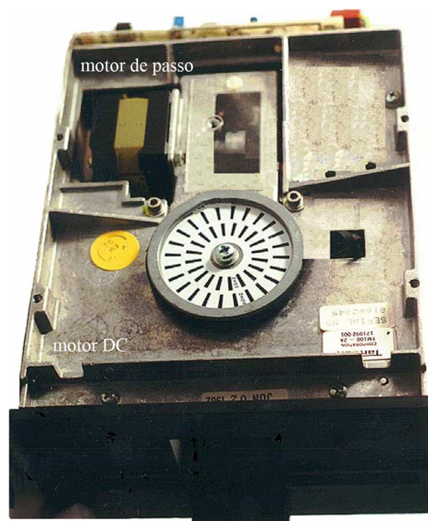
Figura 1 - Leitor antigo de disquete de 5.25 polegadas.
