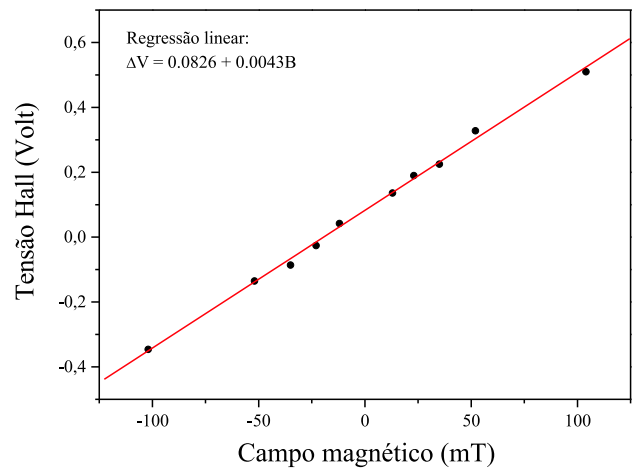
Figura 6 - Calibração do sensor Hall, usando um gaussímetro comercial.
