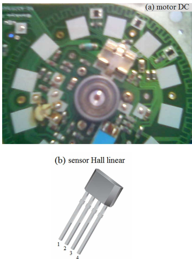
Figura 2 - (a) Motor DC de 5.25 polegadas, contendo 3 sensores de efeito Hall. (b) Sensor de efeito Hall linear com dois canais.
