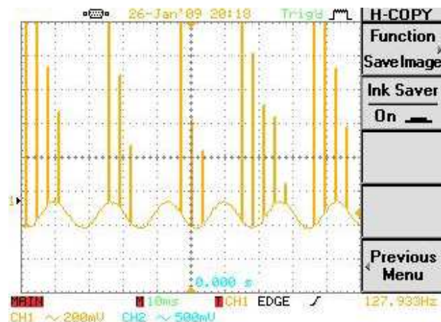
Figura 8 - Saída do CSS, mostrando a superposição do SI com f = 927 Hz e da OS com f = 60 Hz.
