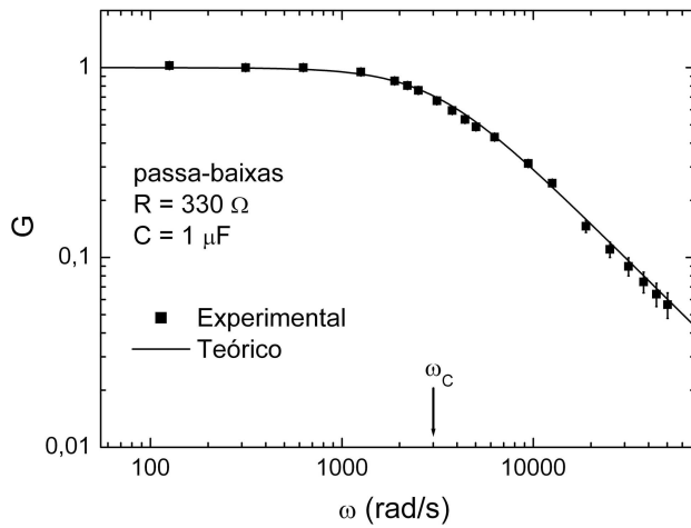
Figura 5 - Ganho em função da frequência angular para um filtro passa-baixas com R = 330 \Omega e C = 1 \mu\text{F} . A linha sólida representa a função correspondente ao ganho dado pela Eq. (3).
