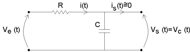
Figura 1 - Modelo de um circuito RC com tensão de saída medida no capacitor.
