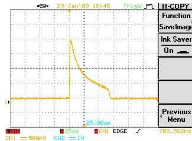
Figura 3 - Detalhe do SI com escala de tempo expandida, mostrando a parte do sinal correspondente à descarga do capacitor.
