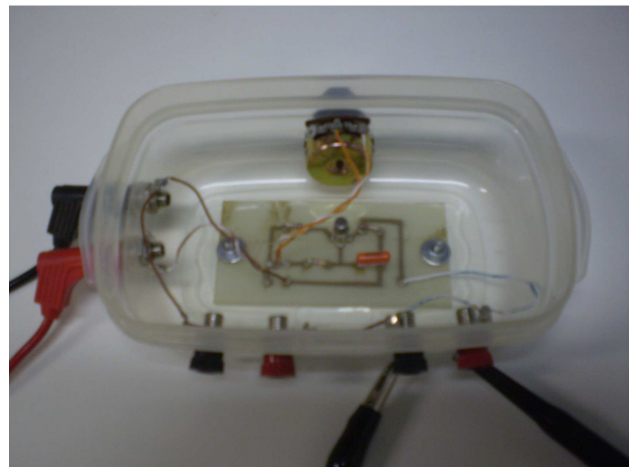
Figura 2 - Esquema do CSS (acima), foto do pote plástico que abriga os conectores para que possa ser realizada a superposição de sinais (centro) e detalhe do circuito no interior do pote plástico (abaixo). A entrada E recebe a onda senoidal e a saída S fornece o resultado da superposição. Na parte traseira está colocado o potenciômetro para variação da frequência do sinal gerado internamente e na lateral, à esquerda, os conectores para a fonte de alimentação.
