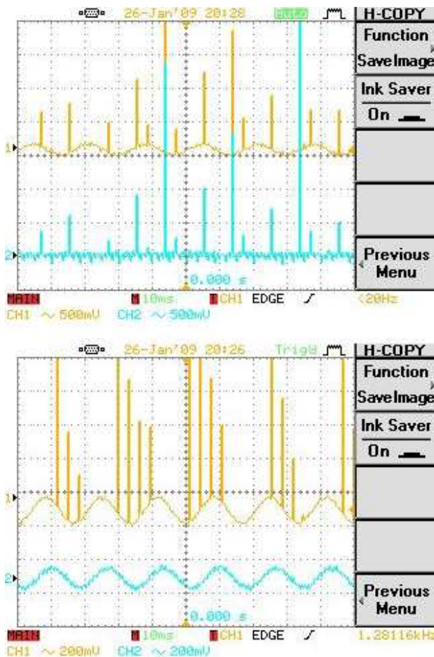
Figura 10 - Acima, entrada e saída do filtro RC para a situação I) (eliminação da OS). Abaixo, entrada e saída do filtro RC para a situação II) (eliminação do SI).
