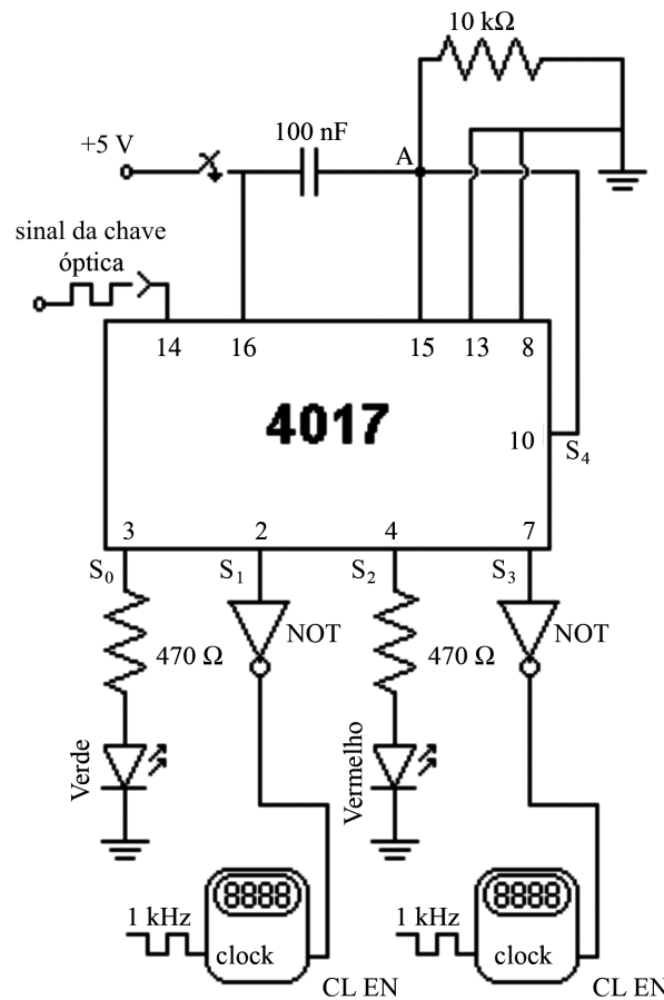
Figura 7 - O CD4017 configurado para acionar seqüencialmente dois contadores.
