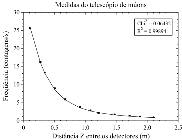
Figura 4 - Comportamento da freqüência de múons com a distância ( Z ) entre os detectores.
