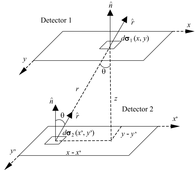
Figura 3 - Desenho da geometria do arranjo de detectores empregado para determinação da abertura do telescópio de múons.
