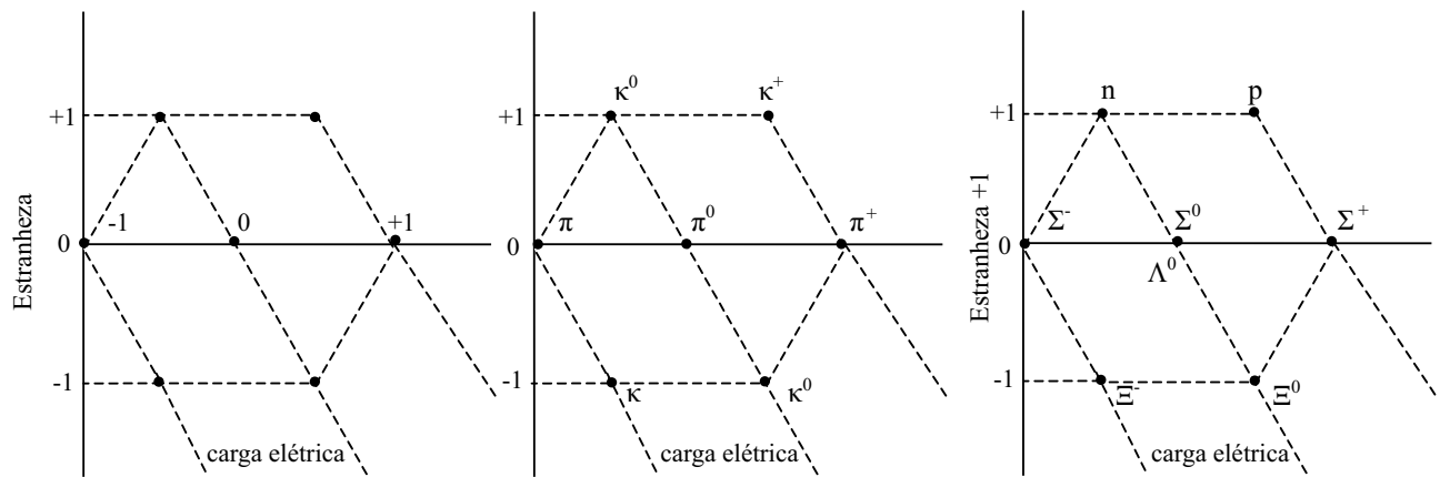
Figura 1 - Padrões hexagonais para mésons e bárions, a partir das propriedades estranheza e carga elétrica, constituindo o chamado caminho óctuplo. A descoberta do méson eta ( \eta^0 ), em 1961, deixou idênticos os dois padrões. 15
