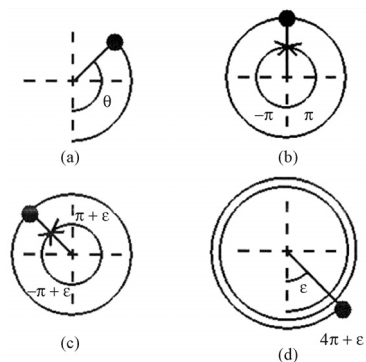
Figura 7 - (a) Orientação do ângulo \theta ; (b) Correspondência entre os ângulos -\pi e \pi ; (c) Correspondência entre um ângulo positivo e maior que \pi e um ângulo negativo menor que -\pi ; (d) Ângulo qualquer maior que 2\pi e seu correspondente no intervalo [-\pi, \pi] .
