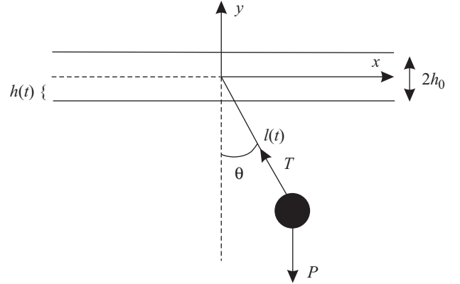
Figura 2 - Representação esquemática de um pêndulo paramétrico com ponto de sustentação oscilante.
