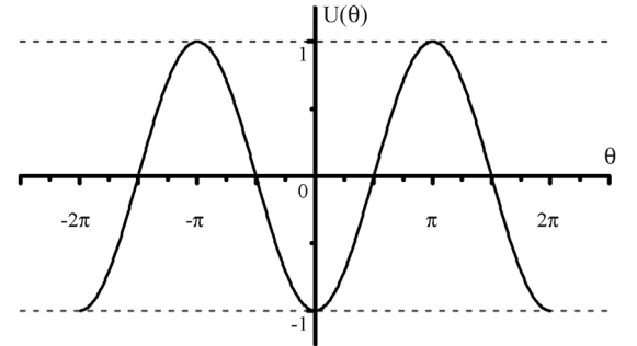
Figura 3 - Potencial U(\theta) = -\cos(\theta) do pêndulo simples.
