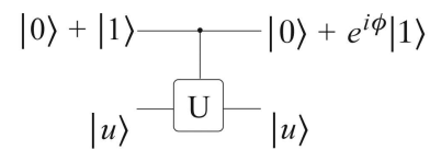
Figura 9 - circuito de computação da fase.
