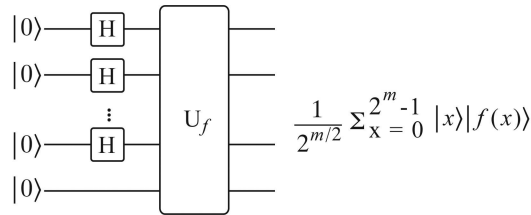
Figura 6 - Computando valor de f para todos os valores de x .
