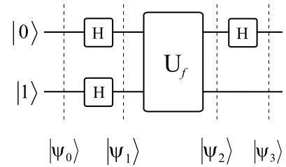
Figura 7 - Circuito de Deutsch.
