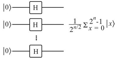
Figura 5 - Circuito que põe registrador no estado \frac{1}{2^{m/2}} \sum_{x=0}^{2^m-1} |x\rangle .
