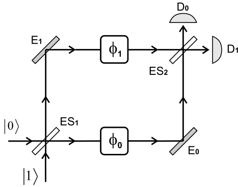
Figura 8 - Visão esquemática do interferômetro de Mach-Zehnder.
