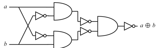
Figura 2 - Circuito que computa a função adição módulo 2.
